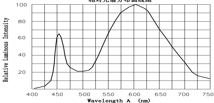
Wavelength Characteristics T_a = 25^\circ\text{C} 相对光谱分布曲线图
