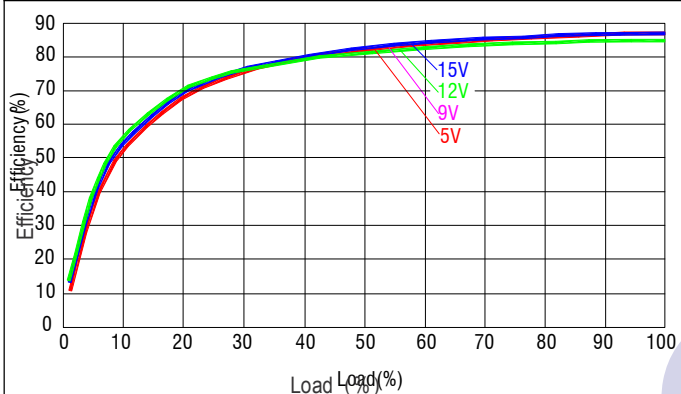
TPNA 48V INPUT VOLTAGE
