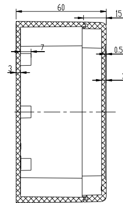
剖面 A-A
