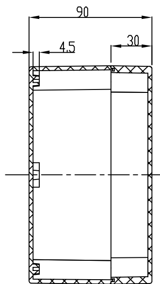
B-B
