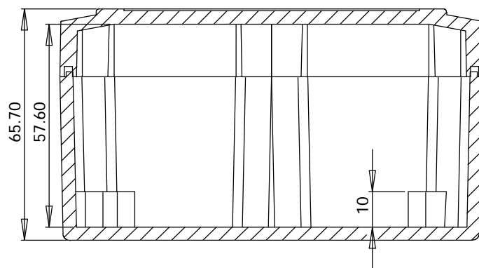
剖面 A-A
