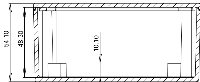
剖面 A-A
