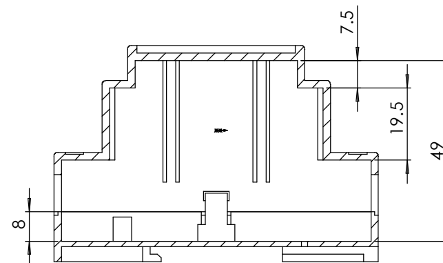
剖面 A-A
