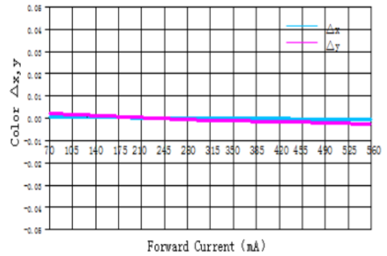
Forward Current vs. Color Δx, y 电流与色坐标偏移量曲线关系
