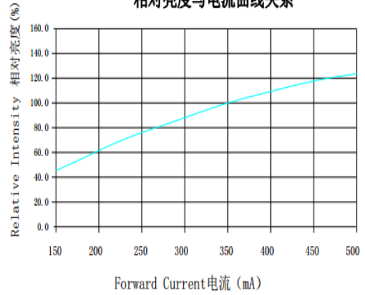
Relative Luminous Flux vs. Forward Current 相对亮度与电流曲线关系
