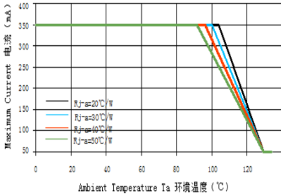
Thermal design 电流与环境温度曲线关系
