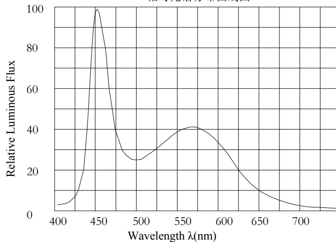
相对光谱分布曲线图
