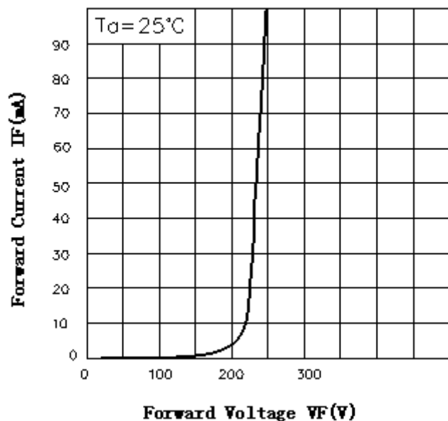
IF - VF 伏安特性曲线图
